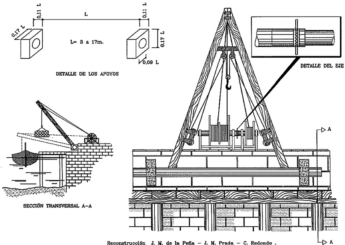
Reconstrucción de grúa portuaria romana de eje horizontal 29 .
